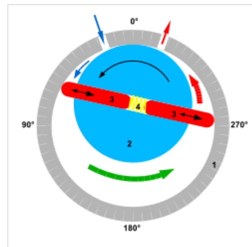
Шибера насос
