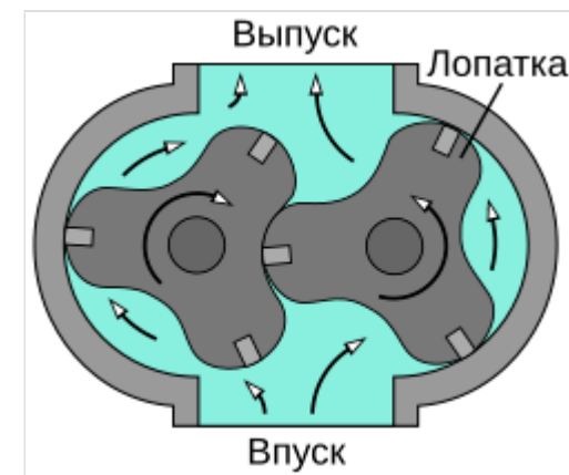
Кулачковый компрессор
